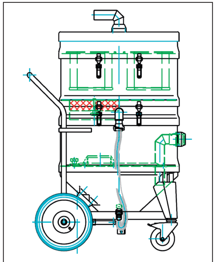
NA 35 modèle WSP - groupe d'aspiration à part
