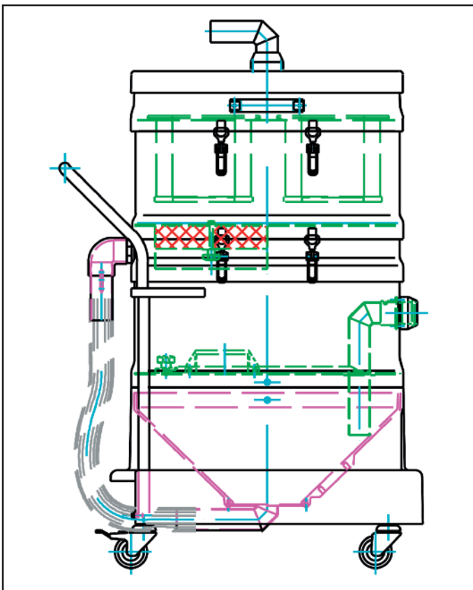
NA 35 modèle DS 1 - groupe d'aspiration à part
