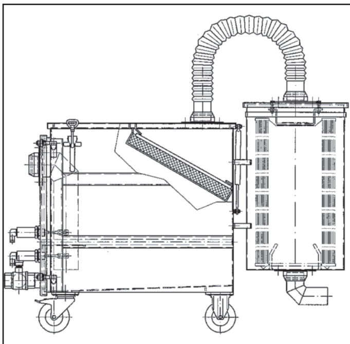
NA 250 type III inox sans filtre supplémentaire
